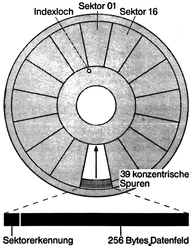
Spuren- und Sektorenlage bei 5.25" Diskette*
